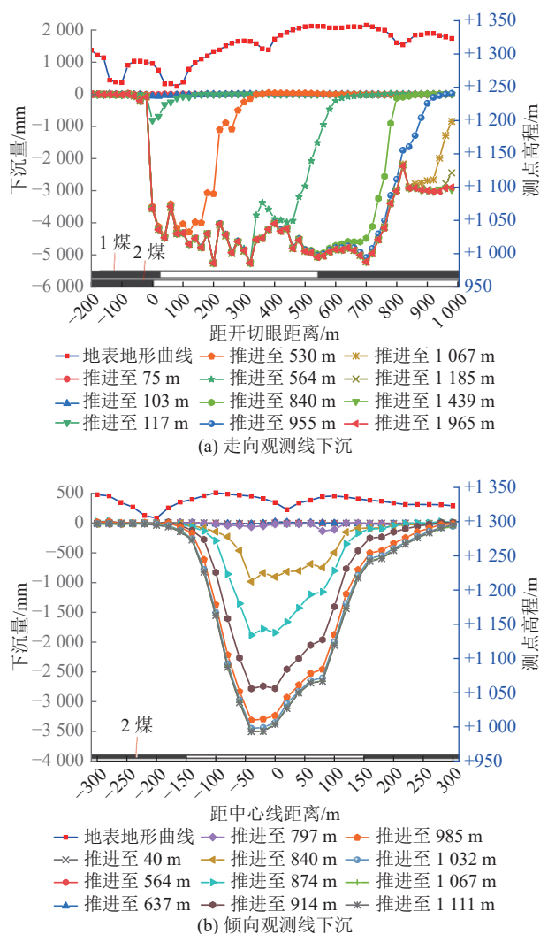
图 2 地表下沉曲线
