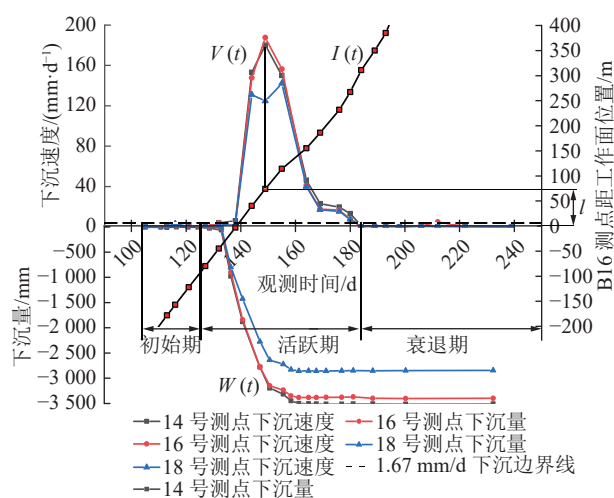
图7 B14、B16、B18号点下沉速度、下沉量与观测时间关系
