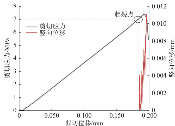
图 10 剪切应力-位移曲线
