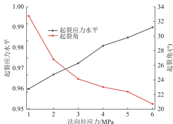
图 11 起裂应力水平及起裂角
