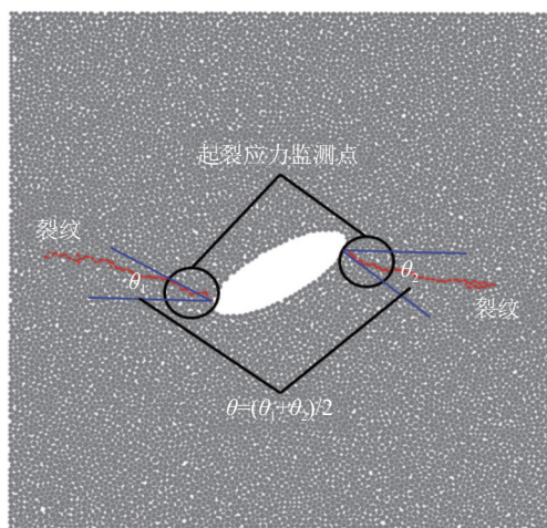
图 9 起裂应力及起裂角监测
