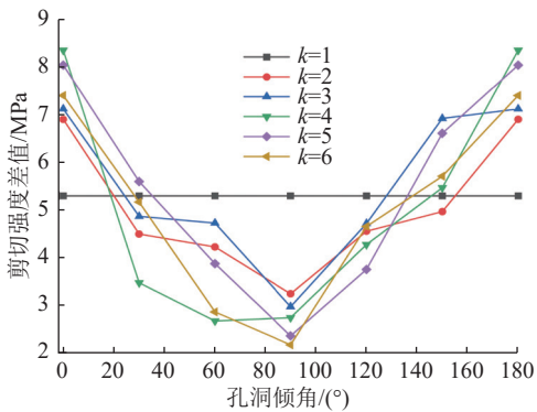
图7 剪切强度差值
