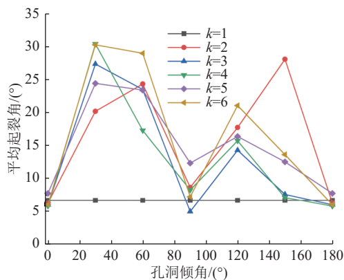
图 12 平均起裂角
