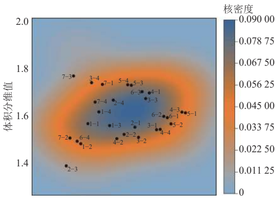
图 12 复合岩层体积分维值核密度 Fig.12 Volume fractal dimension value nuclear density of composite strata
