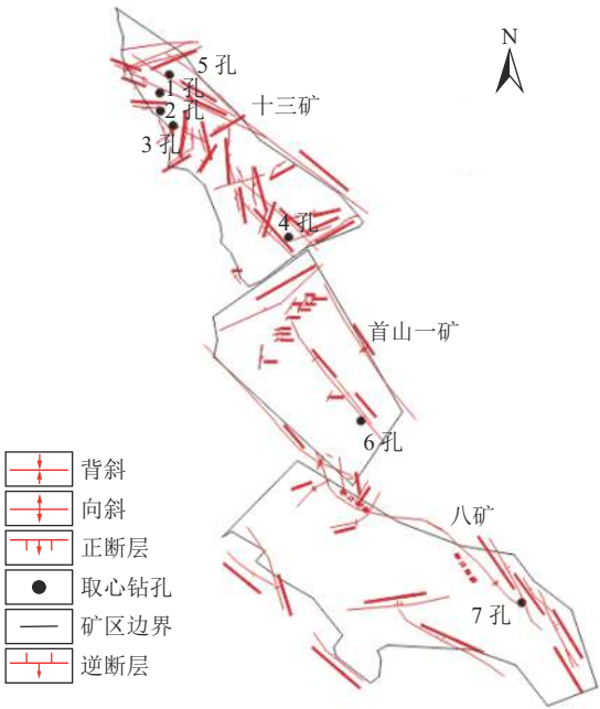
图 2 钻孔位置 Fig.2 Drilling position
