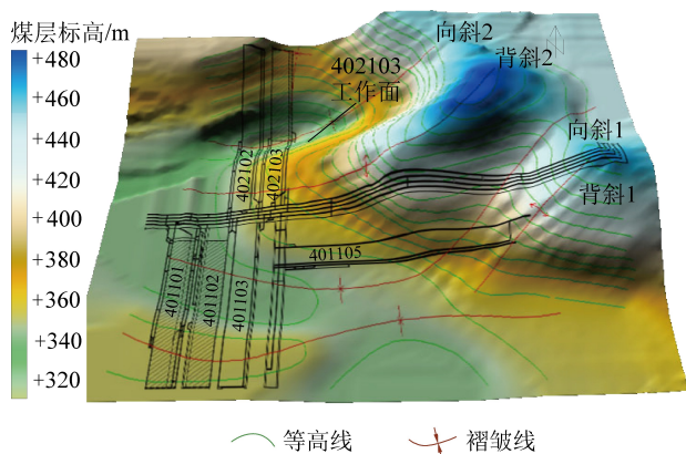
图1 煤矿褶皱构造形态
