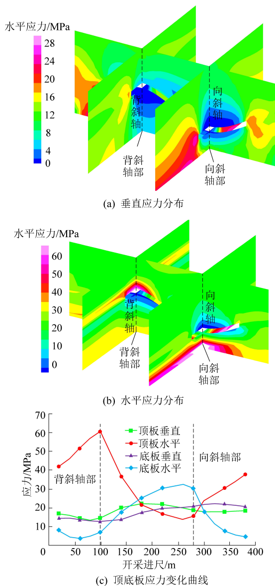
图4 褶皱构造区开采期间顶底板岩层应力演化特征
