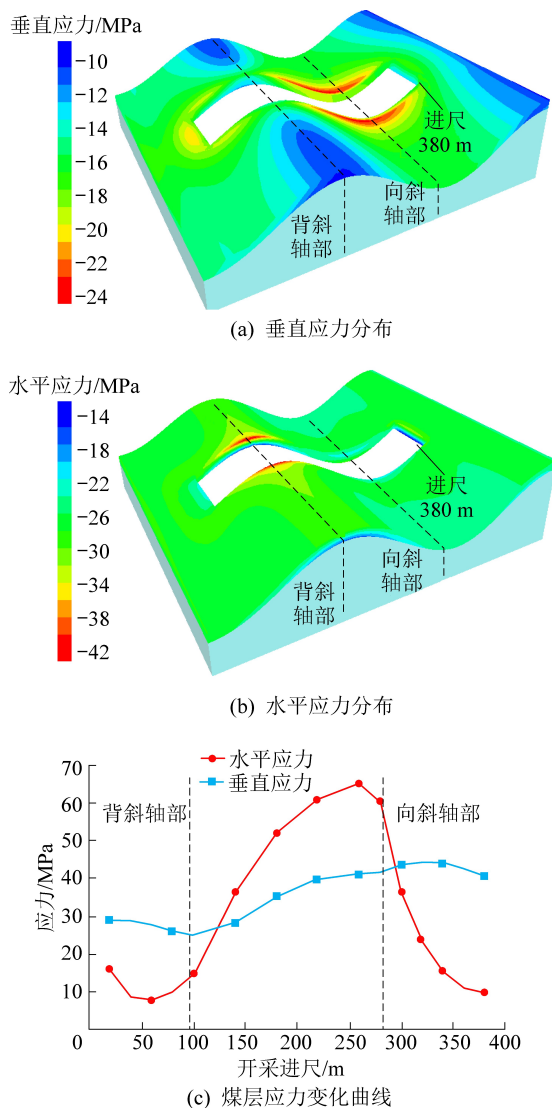
图5 褶皱构造区开采期间煤层应力演化特征
