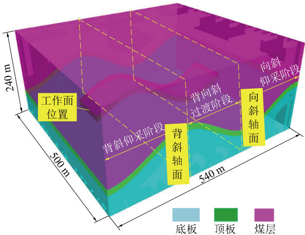
图3 褶皱构造数值计算模型
