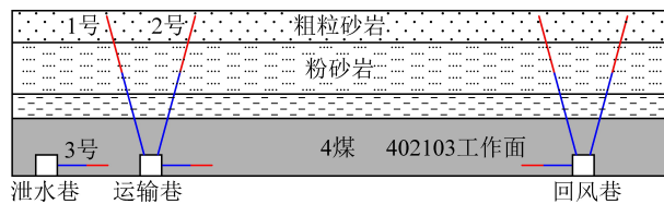
图6 巷道围岩爆破卸压方案示意
